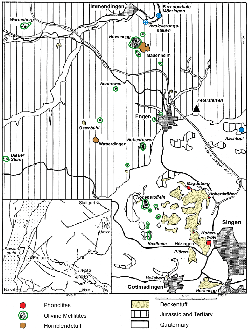
Abb. 13: Vereinfachte geologische Karte der Vulkanitvorkommen im Hegau (verändert nach Keller et al. 1990 und Schreiner 1992)
