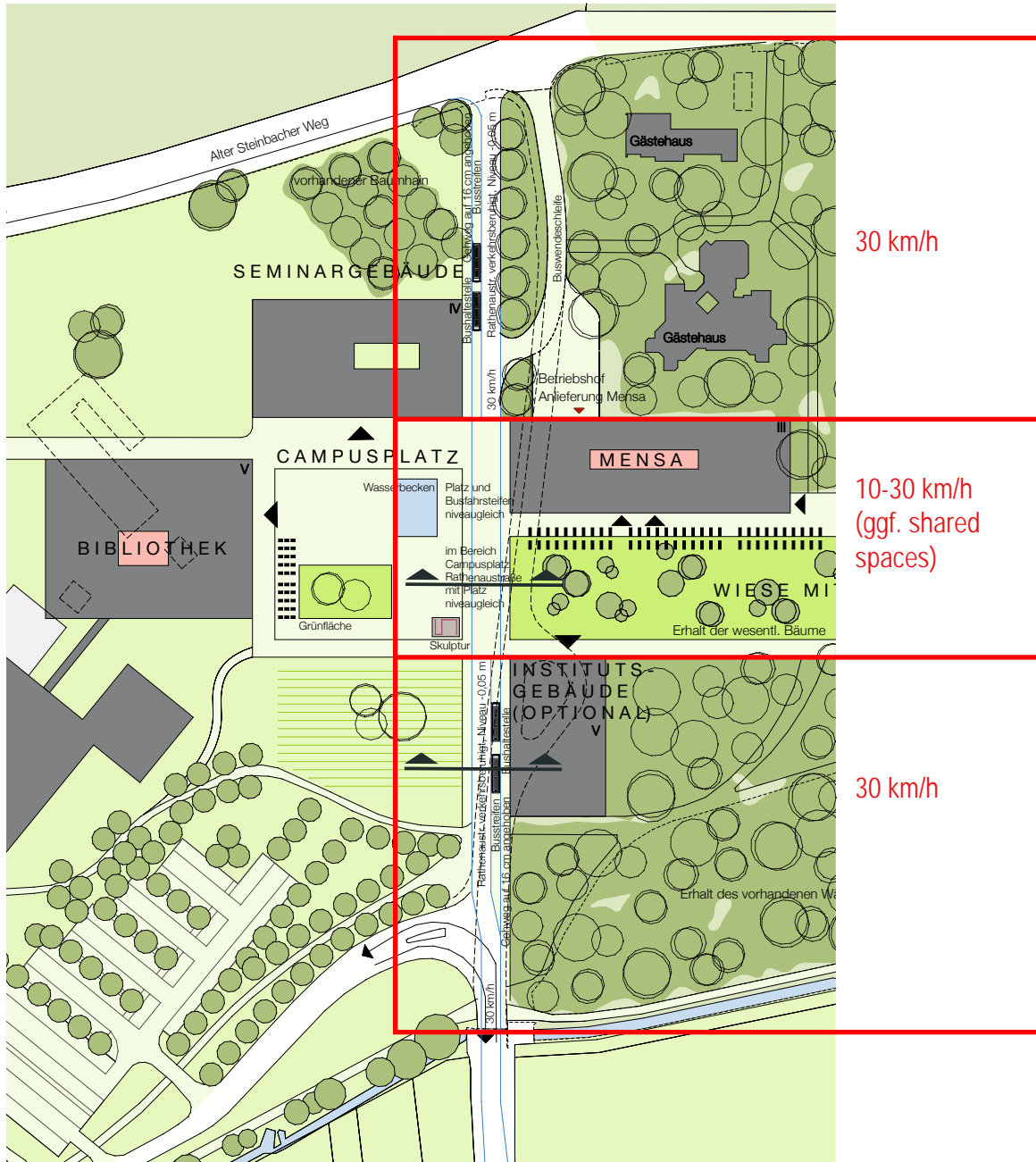
5.2 Verkehrsplanung - Ausbaustufe 2020 - Konzept Rathenaustraße / Campusplatz
