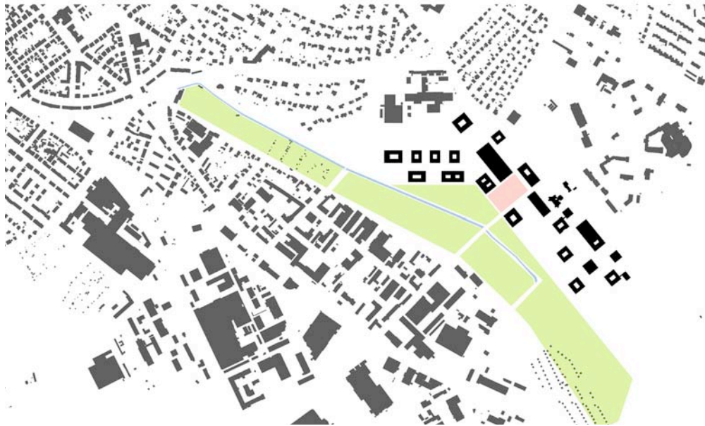
Schwarzplan
