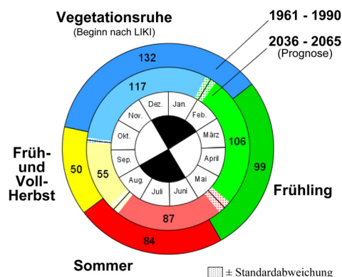
Vereinfachte doppelte phänologische Uhr mit beobachteten und prognostizierten mittleren Eintrittsterminen für das Marburg-Gießener-Lahntal
