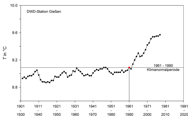
Gleitendes 30jähriges Mittel der Lufttemperatur ( T_m ) in Gießen
