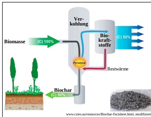
Abb. 2: Schema der C-Sequestrierung mittels Pyrolyse-Biochar: Etwa die Hälfte des Kohlenstoffs der Biomasse wird in Form von Biochar ausgekoppelt und in Böden eingebracht; die anderen 50% werden energetisch oder stofflich genutzt (Syngase oder Bioöle). Denkbar ist auch eine am Markt orientierte Nutzung des Biochars: je nach Marktlage als ( \text{CO}_2 -neutraler) Brennstoff oder als Bodenverbessernder, C-speichernder Bodenhilfsstoff. (Quelle: CSIRO, Australien)
