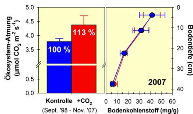
Mittlere Ökosystem-Atmung des Grünlands über das gesamte Experiment (links); Bodenkohlenstoff nach 9,5 Jahren (rechts)
