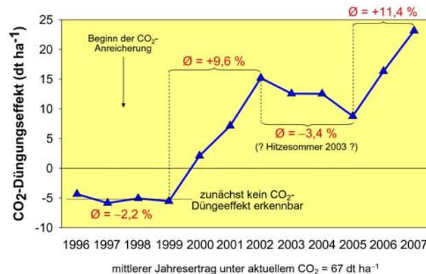
Einfluss des kumulierten CO 2 -Düngereffekts auf die Ertragsleistung (in dt/ha)
