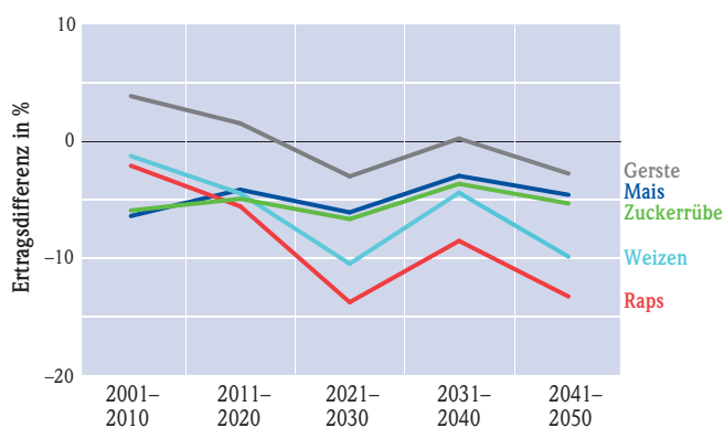
Ertragsänderungen in Hessen relativ zu 1980–2000.
