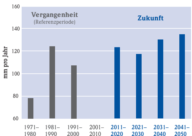
Grundwasserneubildung in Hessen.
